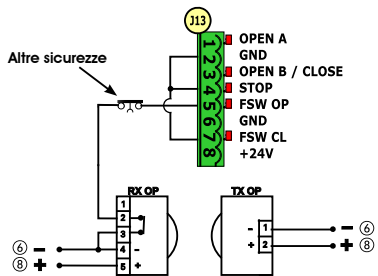
Collegamento una coppia di fotocellule in apertura
