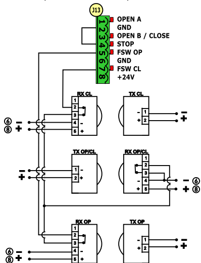
Collegamento di una coppia di fotocellule in chiusura, una in apertura ed una in apertura/chiusura
