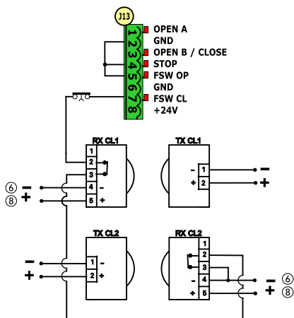
Collegamento di due coppie di fotocellule in chiusura
