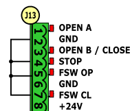
Collegamento di nessun dispositivo di sicurezza e stop
