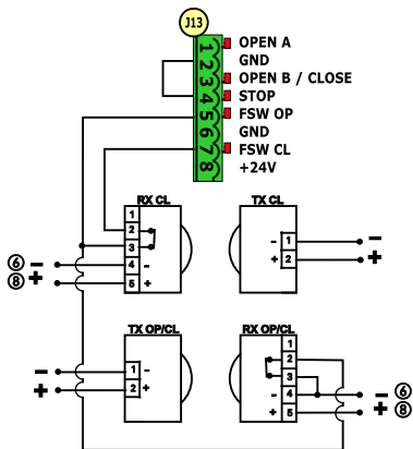
Collegamento di una coppia di fotocellule in chiusura ed una in apertura/chiusura
